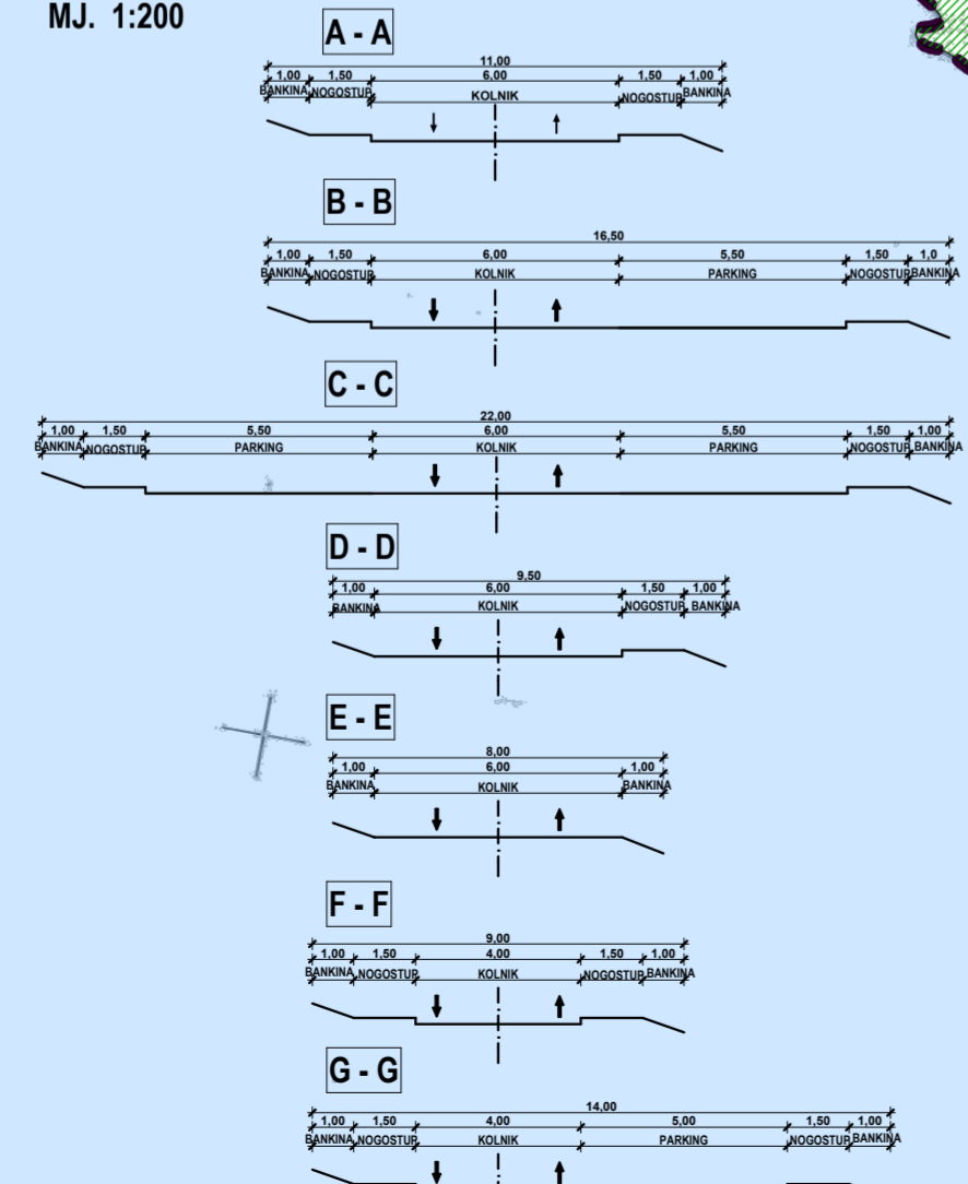
POPREČNI PROFILI CESTOVNE MREŽE M.J. 1:200
